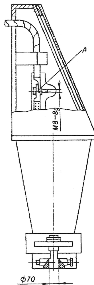
Рис. 4. Коробка выводов с кабельной муфтой для двигателей напряжением 10000 В
