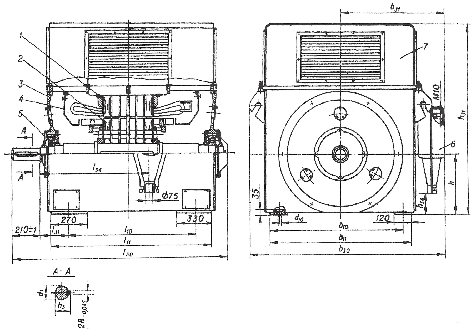
Рис. 1. Асинхронные электродвигатели типа А4
