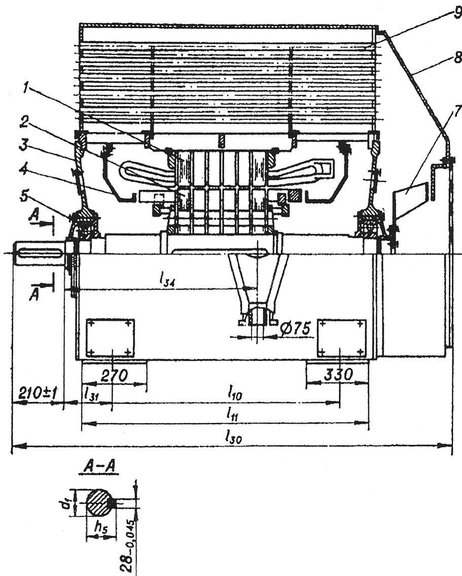
Рис. 3. Асинхронные электродвигатели типа ДАЗО4
